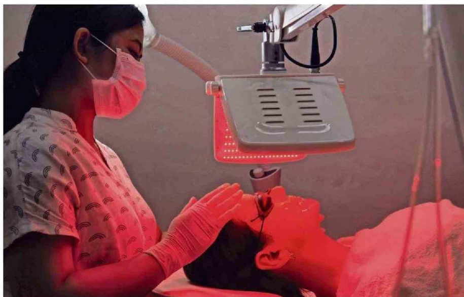
LOS DIODOS EMISORES DE LUZ (LED) TIENEN DIFERENTES LONGITUDES DE ONDA QUE DERIVAN EN COLORES.
