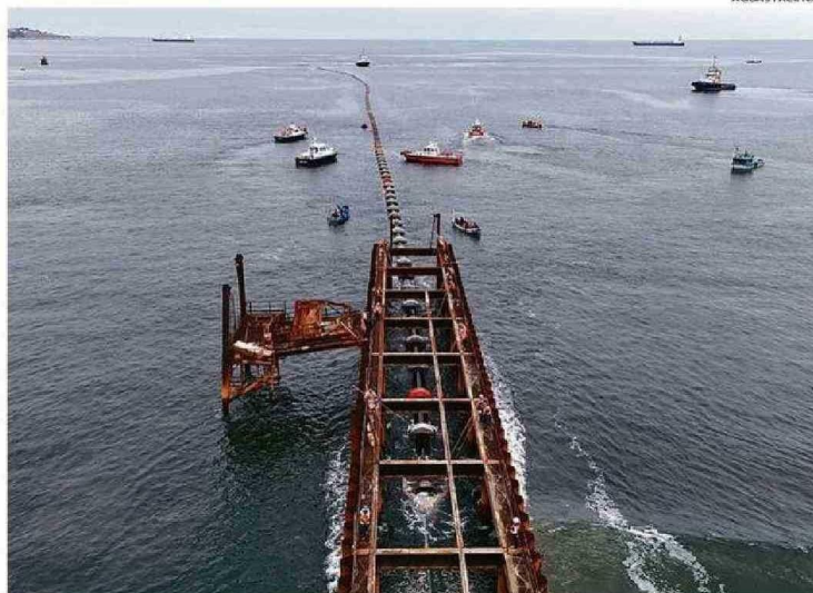
LA EMPRESA REALIZÓ LANZAMIENTO Y HUNDIMIENTO DE LA TUBERÍA DEL EMISARIO EN LA PLANTA.
