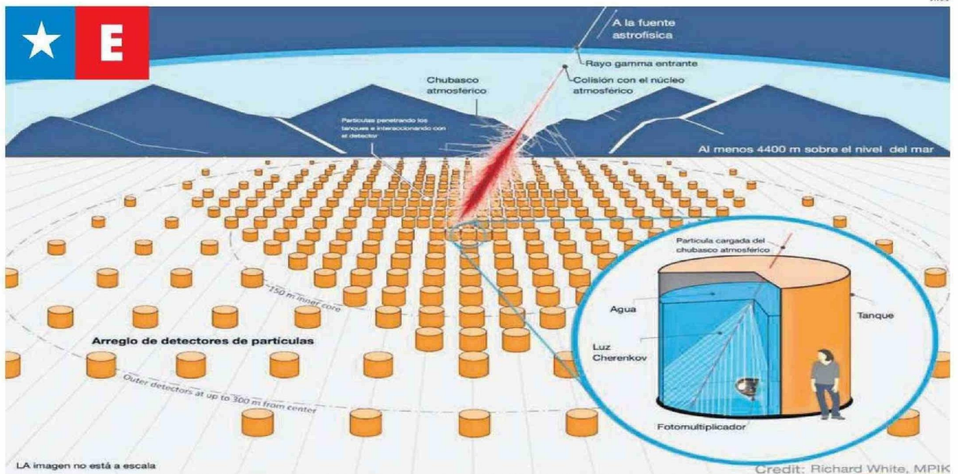
ESTANQUES DE AGUA PURA A 4.700 METROS SOBRE EL NIVEL DEL MAR SERÁN CAPACES DE DETECTAR LA LUZ 'CHERENKOV' Y POR LO TANTO, TRAZAR DESDE QUÉ SECTOR DEL UNIVERSO SE EMITEN RAYOS GAMMA.
