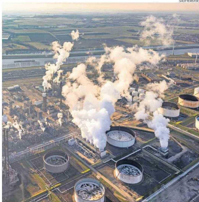
EL CO2 PROCEDE PRINCIPALMENTE DE LA QUEMA DE COMBUSTIBLES FÓSILES Y LA PRODUCCIÓN DE CEMENTO.
