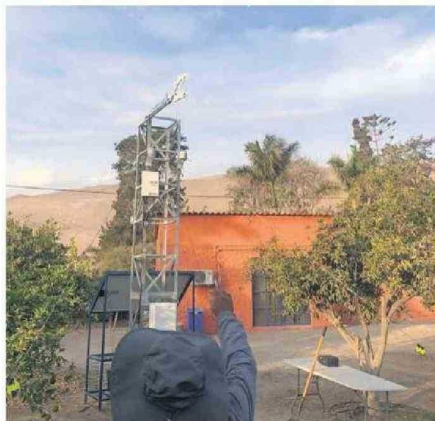
LA TORRE "EDDY COVARIANCE", REALIZARÁ LAS MEDICIONES.
