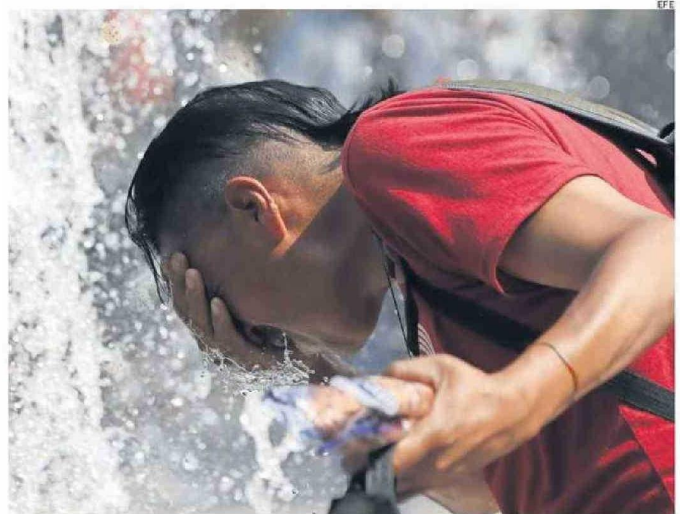
INSTITUCIONES DE TODO EL MUNDO COINCIDIERON EN QUE EL 2024 FUE EL AÑO MÁS CALUROSO DE LA HISTORIA.
