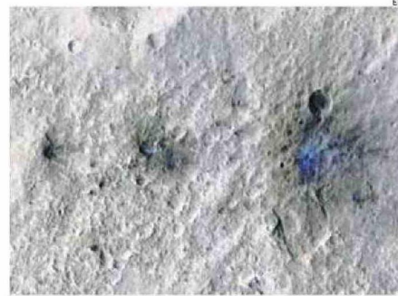
CRÁTERES PRODUCIDOS POR IMPACTOS DE METEORITOS EN MARTE.
