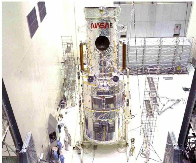
Imagen del telescopio espacial Hubble, antes de su lanzamiento en abril de 1990.
