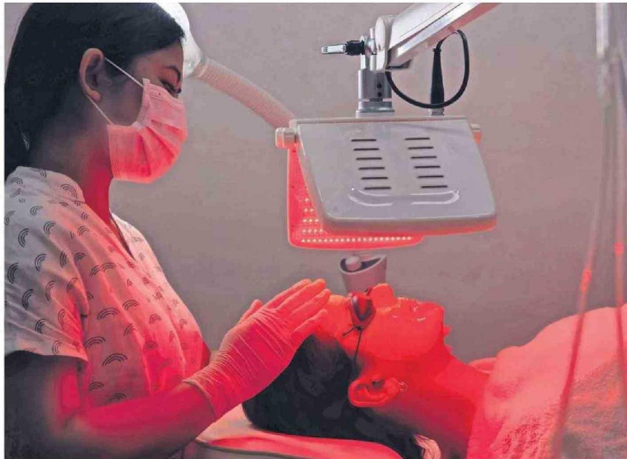
LOS DIODOS EMISORES DE LUZ (LED) TIENEN DIFERENTES LONGITUDES DE ONDA QUE DERIVAN EN COLORES.
