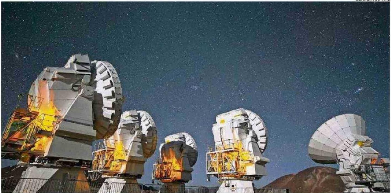
LA OBSERVACIÓN ASTRONÓMICA DESDE EL NORTE CHILENO ES RECONOCIDA COMO LA MEJOR DEL MUNDO.
