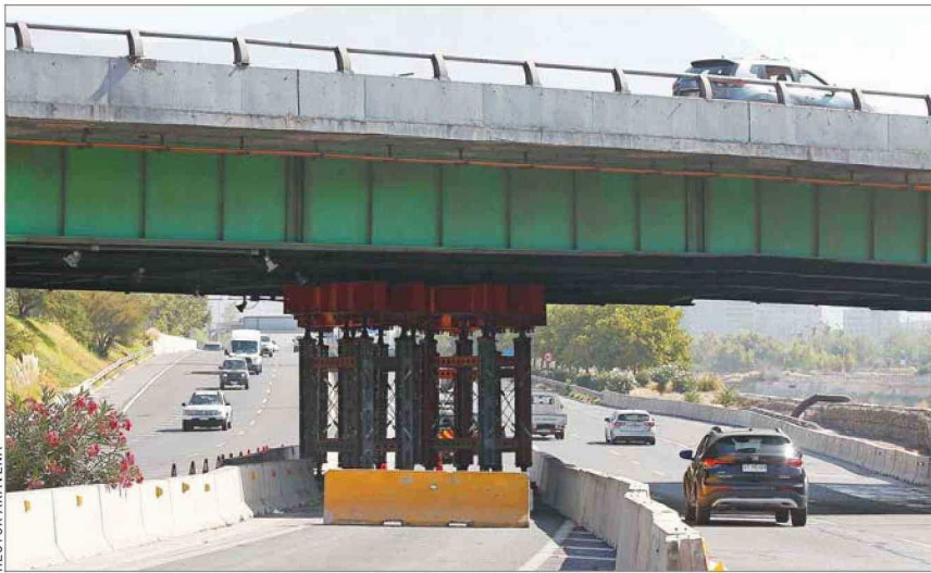
Medida. Torretas fueron instaladas bajo el puente para soportar su peso.
