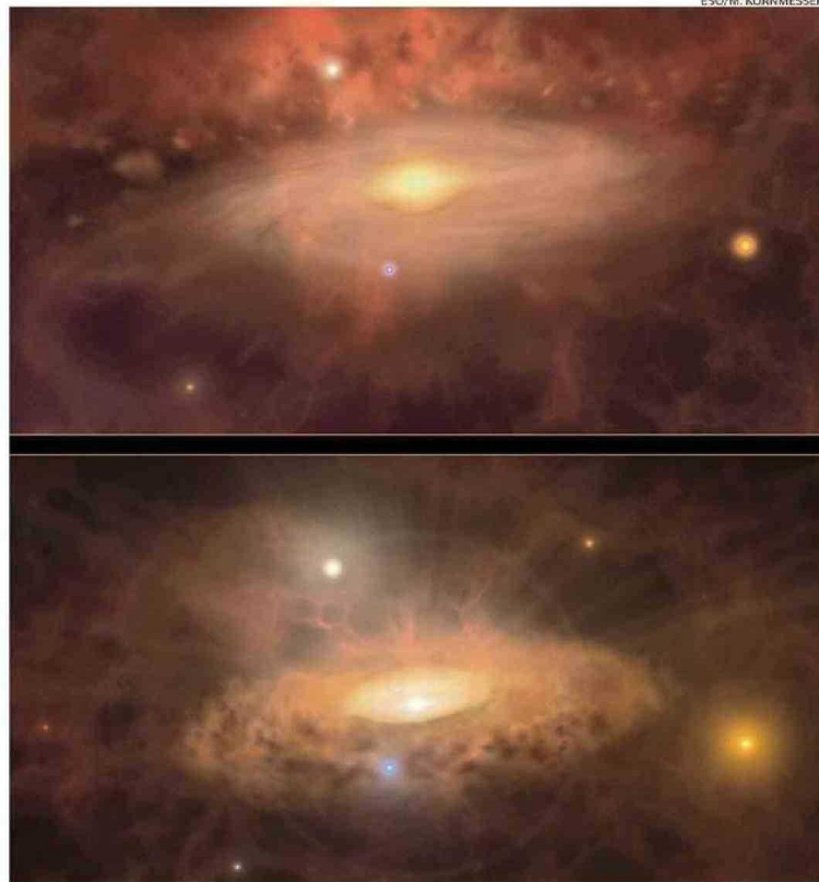
DOS ETAPAS EN LA FORMACIÓN DE DISCO DE GAS Y POLVO ALREDEDOR DE AGUJERO NEGRO AL CENTRO DE UNA GALAXIA.
