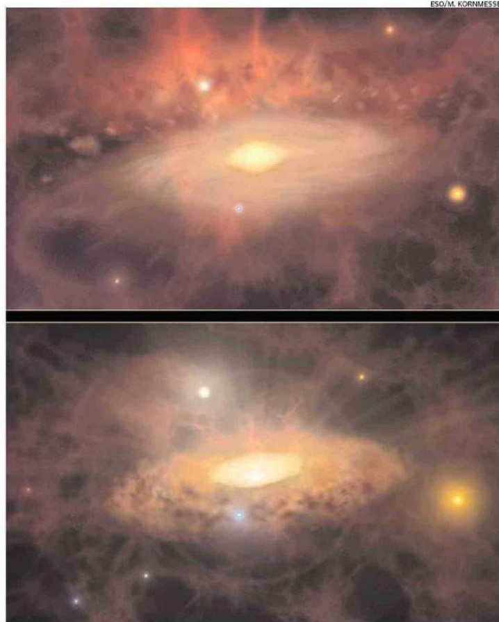
DOS ETAPAS EN LA FORMACIÓN DE DISCO DE GAS Y POLVO ALREDEDOR DE AGUJERO NEGRO AL CENTRO DE UNA GALAXIA.
