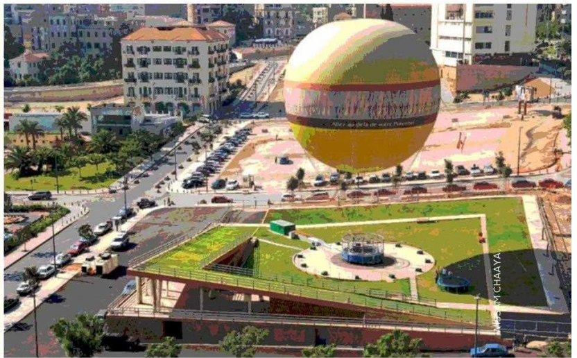
En el centro de Beirut diseñó esta plataforma para un globo de helio, de uso turístico, que saca partido a la pendiente natural del sitio.
