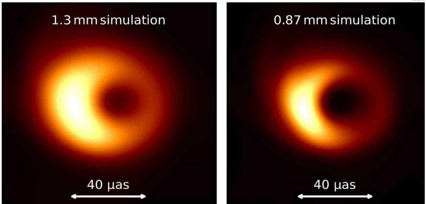
LA IMAGEN SIMULADA ES UNA COMPARACIÓN EN LA IMAGEN DEL AGUJERO NEGRO SAGITARIO A* CON DIFERENTES LONGITUDES DE ONDA. A 0,87 MM LA RESOLUCIÓN ES MAYOR. LA BARRA DE ABAJO INDICA UNA ESCALA ANGULAR DE 40 MICROSEGUNDOS DE ARCO.
