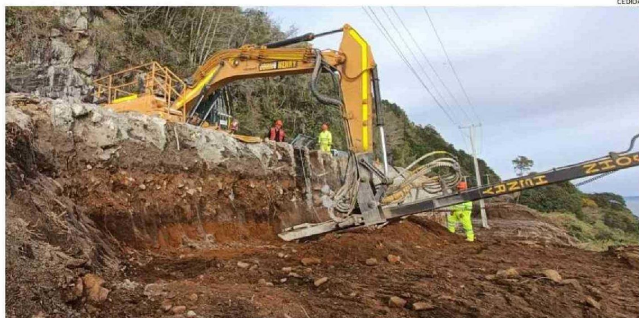
SE CONSTRUYE UN MURO CORTINA DE HORMIGÓN DE SHOTCRETE CON MICROPILOTES, MÁS DOS NIVELES CON PERNOS DE ANCLAJE POSTENSADOS.
