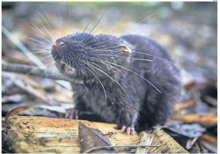
UN RATÓN ANFIBIO (DAPTOMYS SP.) ES UNO DE LOS CUATRO MAMÍFEROS NUEVOS DESCUBIERTOS.
