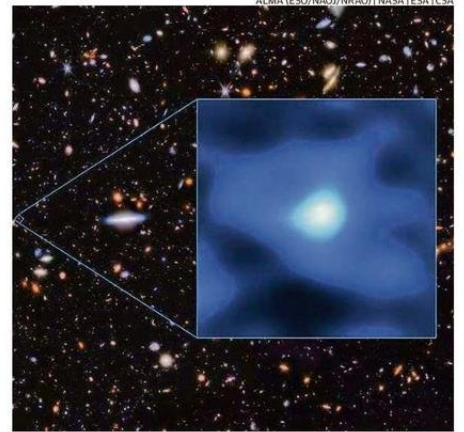
"JADES-GS-z14-0" está a 13.400 millones de años luz de la Tierra.
