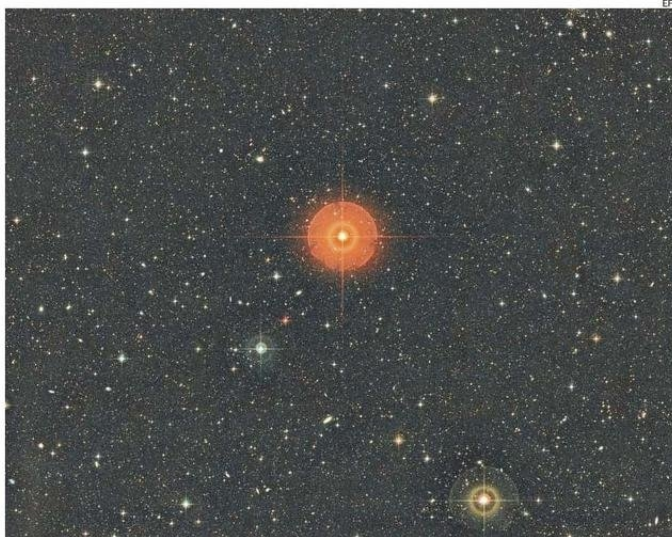
R DORADUS ES LA ESTRELLA DE COLOR NARANJA QUE SE VE EN EL CENTRO DE LA IMAGEN.
