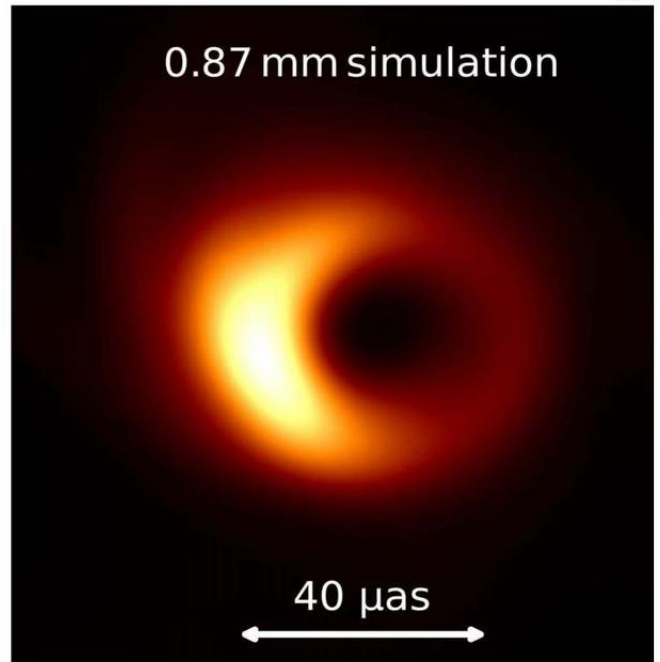
LA IMAGEN SIMULADA ES UNA COMPARACIÓN EN LA IMAGEN DEL AGUJERO NEGRO SAGITARIO A* CON DIFERENTES LONGITUDES DE ONDA. A 0,87 MM LA RESOLUCIÓN ES MAYOR. LA BARRA DE ABAJO INDICA UNA ESCALA ANGULAR DE 40 MICROSEGUNDOS DE ARCO.
