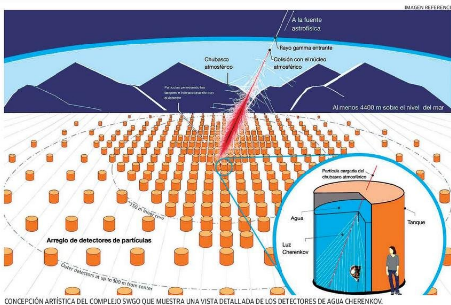
CONCEPCIÓN ARTÍSTICA DEL COMPLEJO SWGO QUE MUESTRA UNA VISTA DETALLADA DE LOS DETECTORES DE AGUA CHERENKOV.
